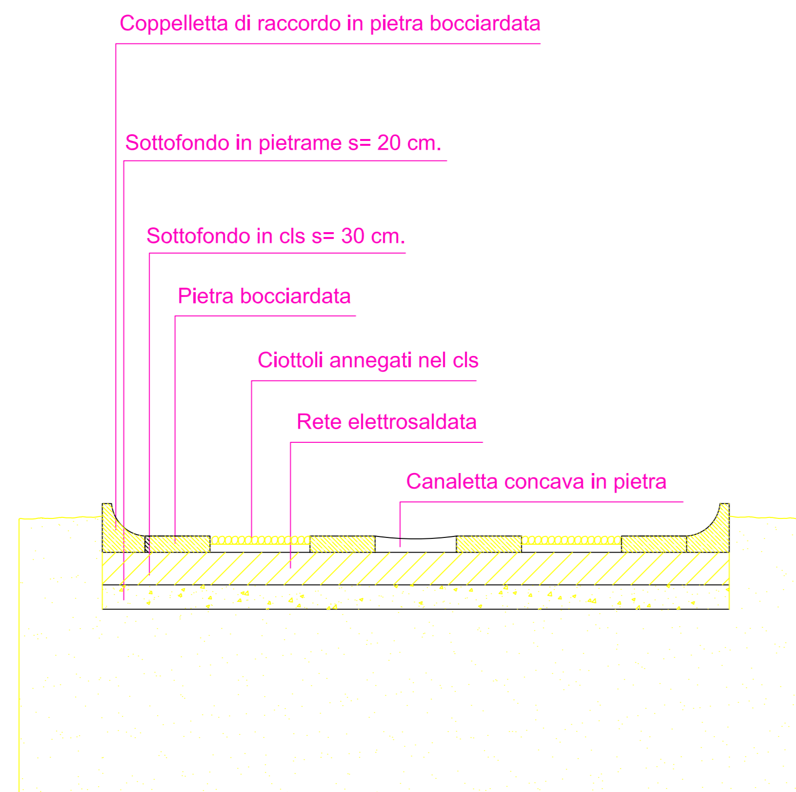
PARTICOLARE SEZIONE STRADALE BB Scala 1:20
